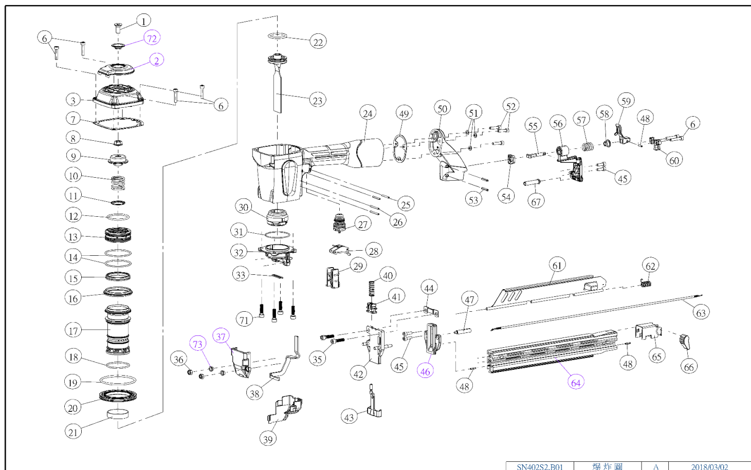
SN402S2.B01 爆炸圖 A 2018/03/02
