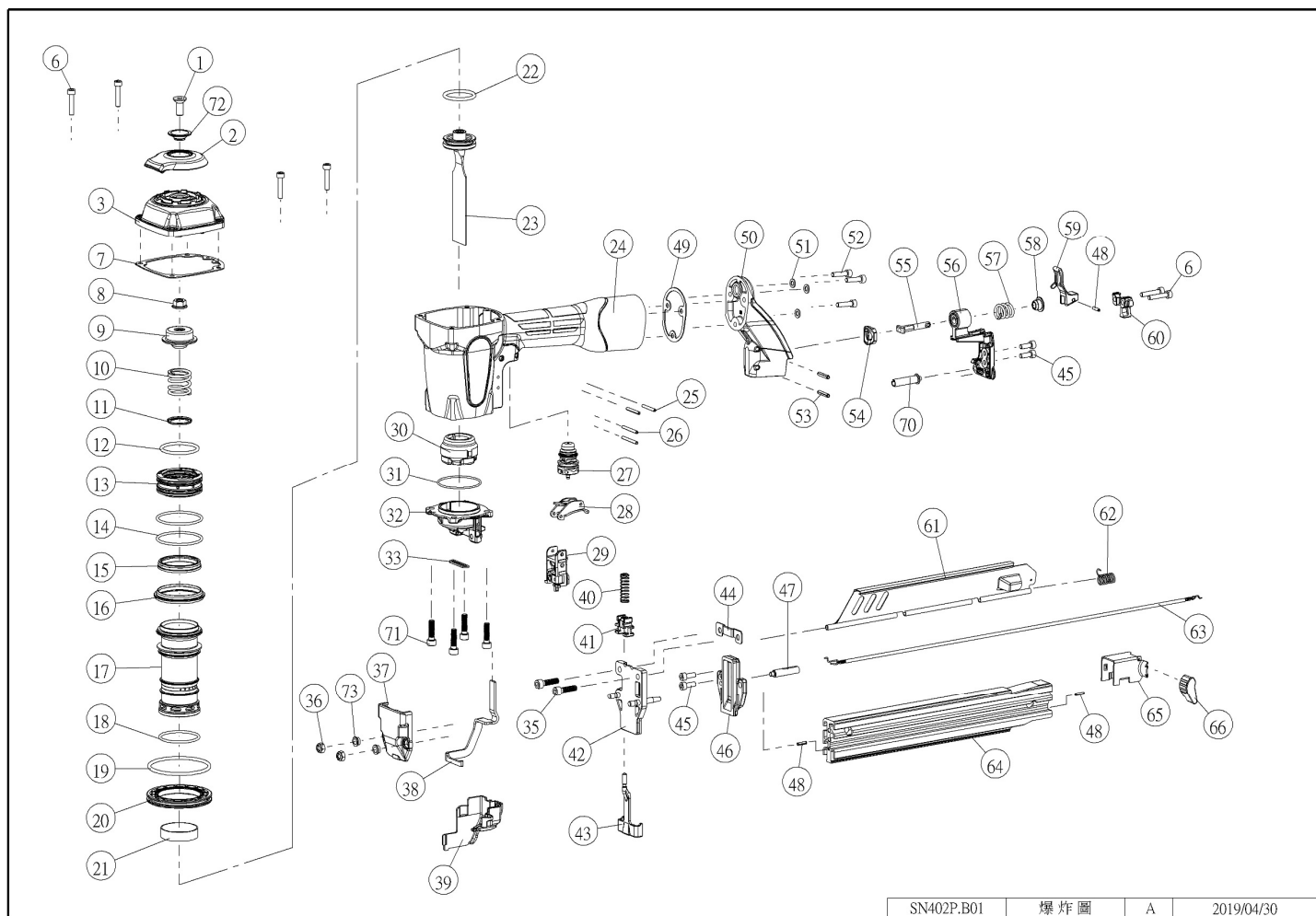
SN402P.B01 爆炸圖 A 2019/04/30
